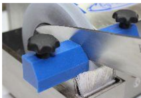
Messerschleifen mit Winkelführung
